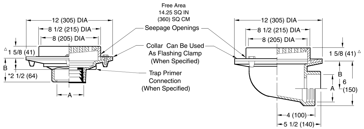
Fig. 2110C ... CAULK OUTLET Fig. 2110Y ... NO-HUB OUTLET
