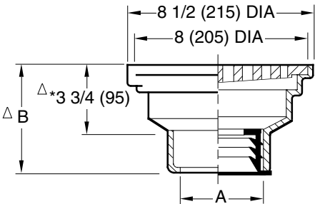
Fig. 2270C ... CAULK OUTLET Fig. 2270Y ... NO-HUB OUTLET
